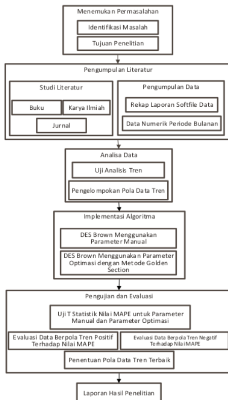
Gambar 1. Metodologi Penelitian
