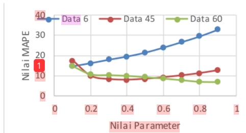
Gambar 3. Grafik Plot Nilai MAPE terhadap nilai parameter untuk beberapa data yang berpola tren negatif.
