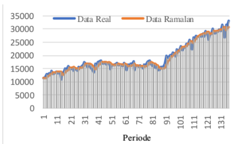
Gambar 4. Plot Perbandingan Data Aktual dengan Data Ramalan pada Data 16
