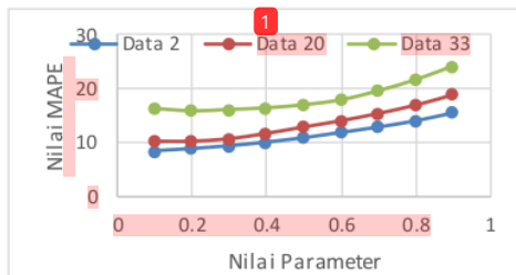
Gambar 2. Grafik Plot Nilai MAPE terhadap nilai parameter untuk beberapa data yang berpola tren positif.
