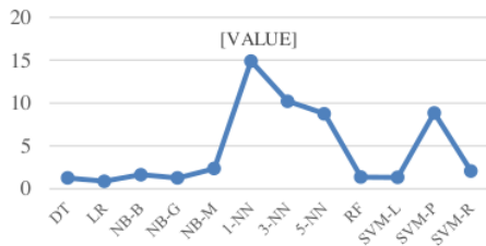
Gambar 4. Grafik gap akurasi
