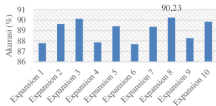
Gambar 3. Perbandingan Akurasi Dataset Expansion
